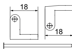
Drehbandsatz
