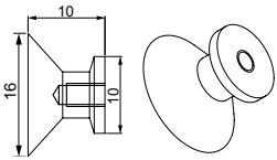
Knopfgriff mit Innengewinde
