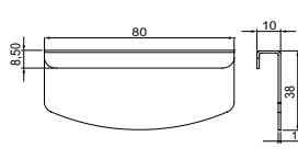
Griffschale
