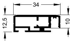
221 Rahmenprofil
