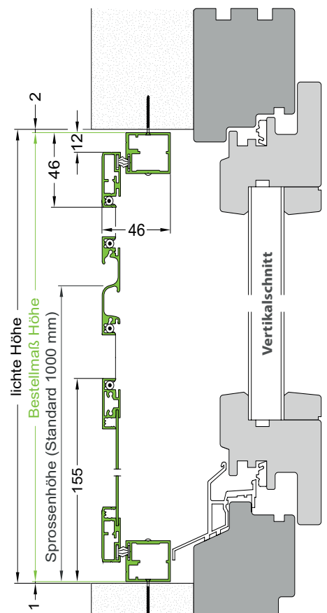
243 Montagerahmenprofil
