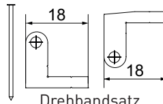
Drehbandsatz
