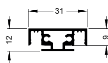
231 Sprosse
