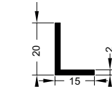
302 Winkelprofil
