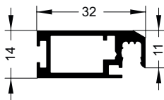
224 Rahmenprofil
