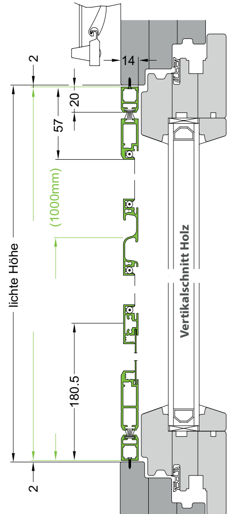
244 Montagerahmenprofil
