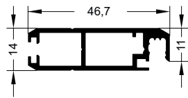
225 Rahmenprofil
