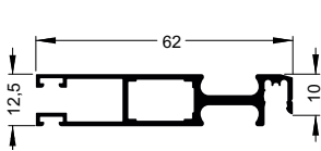
252 Rahmenprofil
