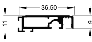
209 Rahmenprofil
